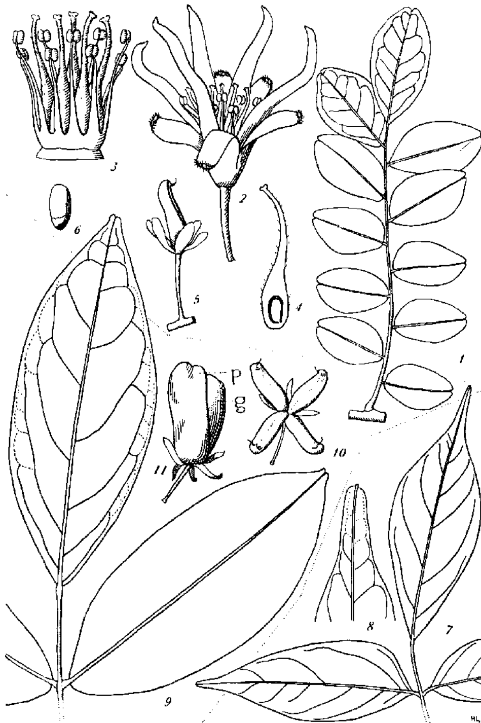
PL. II. — Roureopsis stenopetala : 1, feuille \times 2/3 ; 2, fleur \times 3 ; 3, étamines et pistil \times 6 ; 4, carpelle en coupe \times 6 ; 5, fruit jeune \times 1 ; 6, graine \times 3/2 . — R. emarginata : 7, folioles \times 2/3 ; 8, sommet d'une foliole \times 2 . — R. acutipetala ssp. borneensis : 9, folioles \times 2/3 ; 10, fruits jeunes \times 1 ; 11, fruit mûr \times 1 (p, péricarpe déhiscent, g, graine). — (1, Thorel 3357; 2-4, Poilane 13 263; 5-6, Pierre 906; 7-8, Poilane 13 505; 9, 11, Evrard 591; 10, Poilane 6719).
